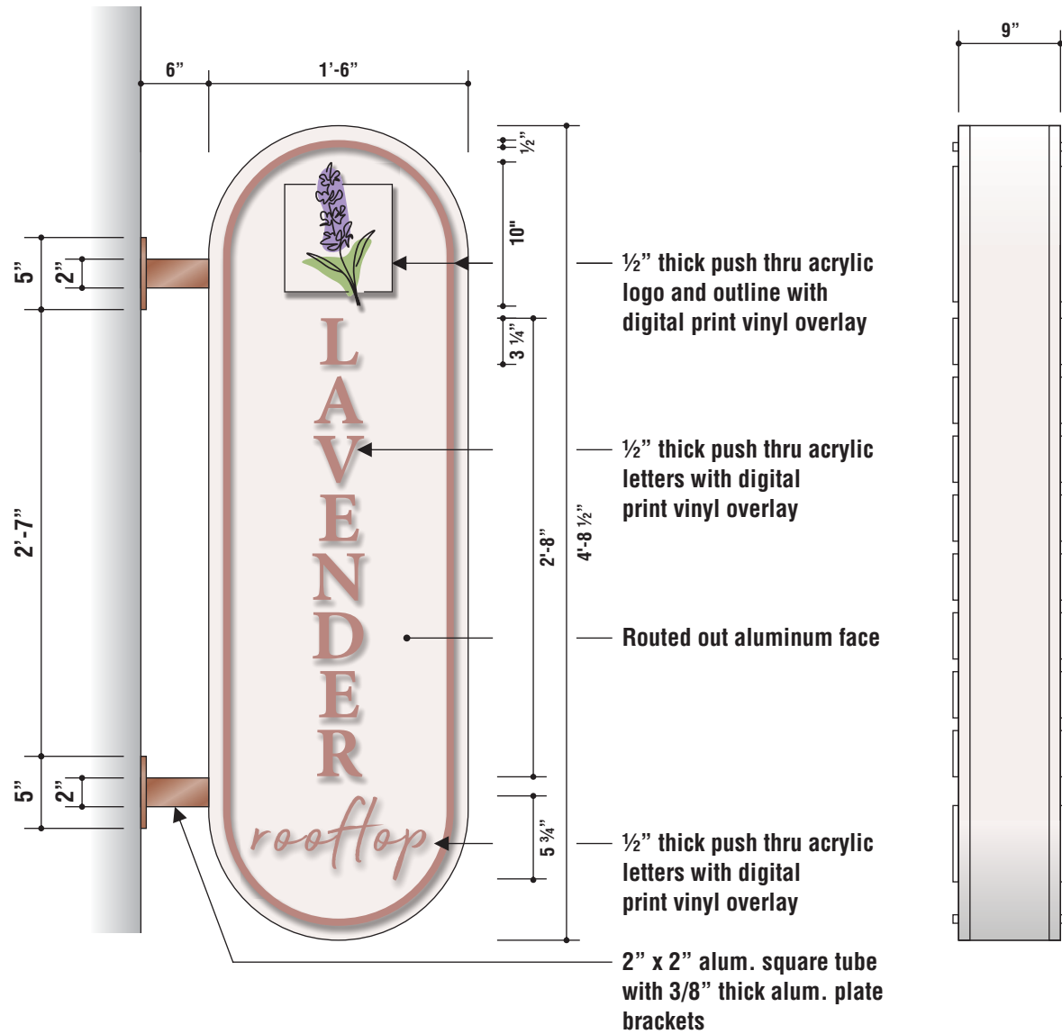
1 Front View Scale: 1" = 1'-0"
